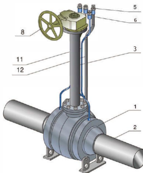
加长杆球阀
