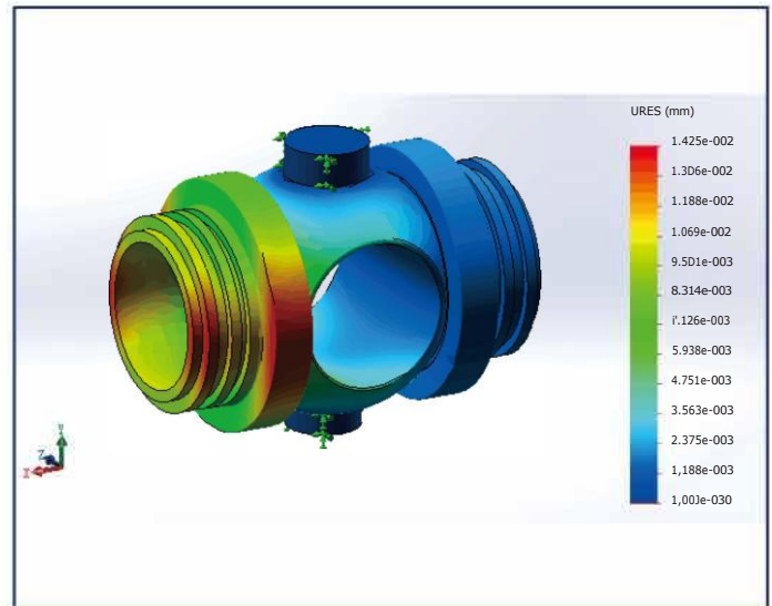
有限元分析
